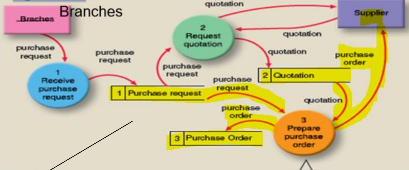
Diagram 0 DFD
